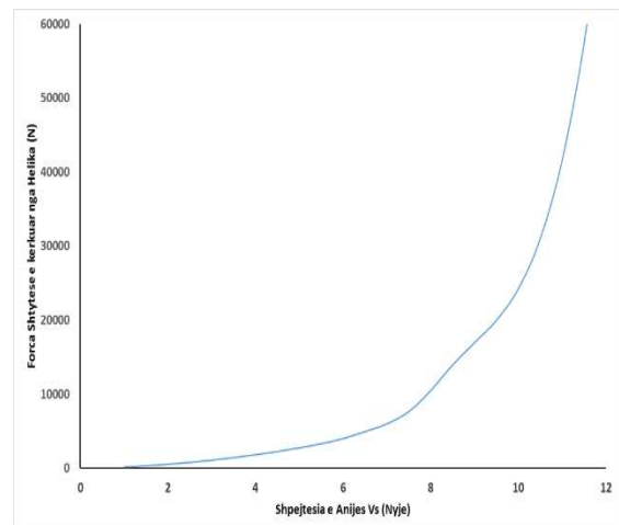
Figura 6. Grafiku i forcës shtytëse të kërkuar nga helika, ndërtuar sipas llogaritjeve të softuerit "Fuqi Anije V 1.0".
