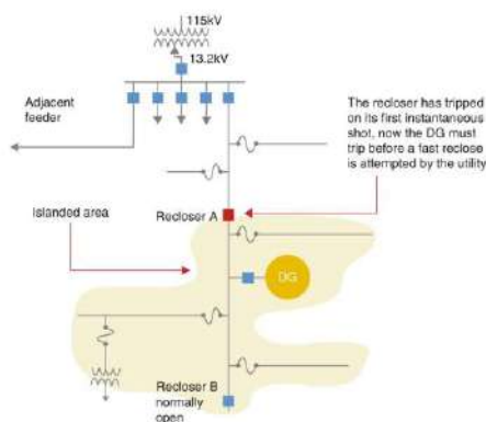
Fig 2: Skema e funksionimit te Microgrids
