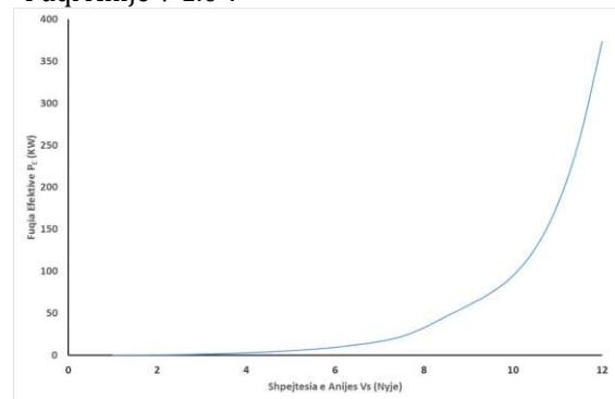
Figura 7. Grafiku i fuqisë efektive, ndërtuar sipas llogaritjeve të softuerit "Fuqi Anije V 1.0".
