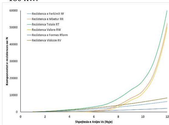
Figura 5. Grafikët e komponentëve të rezistencës, ndërtuar sipas llogaritjeve të softuerit "Fuqi Anije V 1.0".
