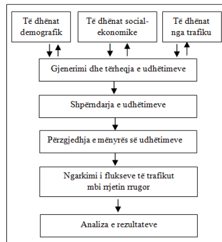
Fig. 1. Ndërtimi skematik i modelit klasik të transportit
