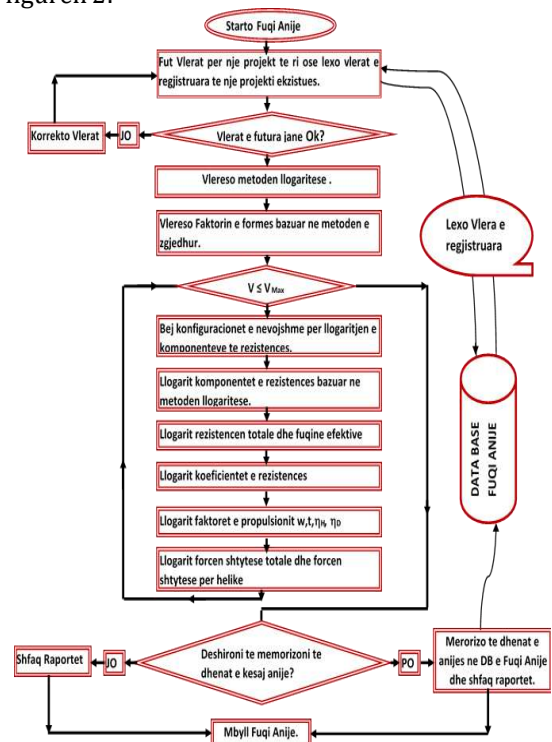
Figura 2. Bllokskema e përgjithshme e softit "Fuqi Anije V 1.0" [7], [9], [13].
