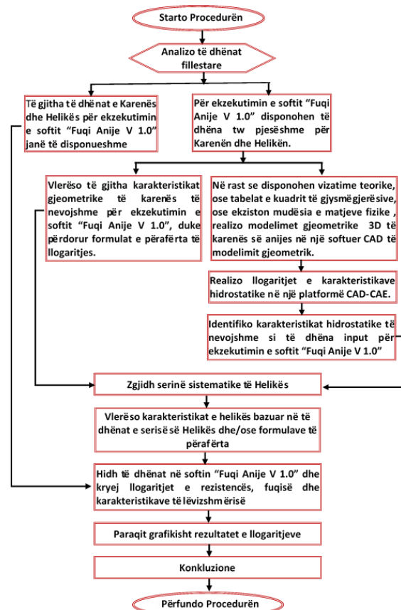
Figura 3. Bllok skema e metodologjisë së studimit.
