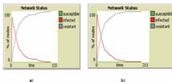
Fig 2.3.4: Paraqitja grafike e numrit të nyjeve në gjendjet susceptible, infectious/infectied, removed/resistant në përfundim të simulimit të SIR në grafën e plotë K_{200} në NetLog. a) Rasti I b) Rasti II .
