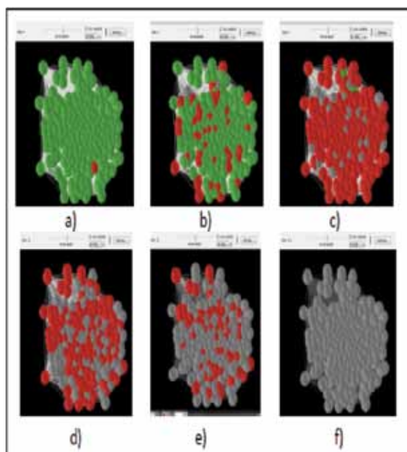
Fig 2.3.4: Paraqitja grafike e numrit të nyjeve në gjendjet susceptible, infectious/infectied, removed/resistant në përfundim të simulimit të SIR në grafën e plotë K_{200} në NetLog. a) Rasti I b) Rasti II .
